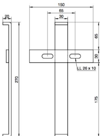
MASTHALTER VARIO-1
