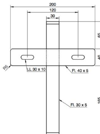
MASTHALTER VARIO-2
